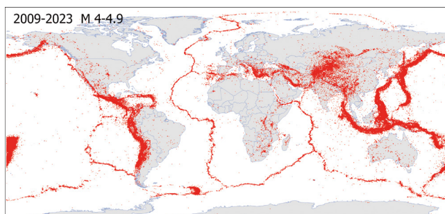
Землетрясения M4,0-4,9 в мире в период 2009-2023 гг.
