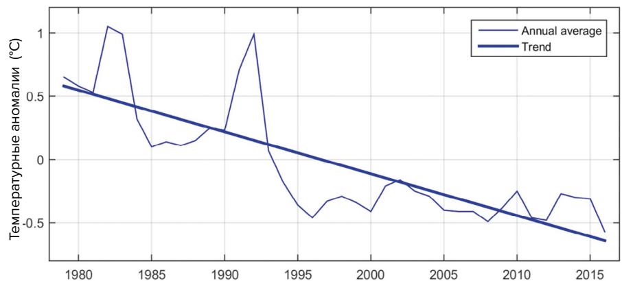
Среднегодовые аномалии глобальной температуры в стратосфере
